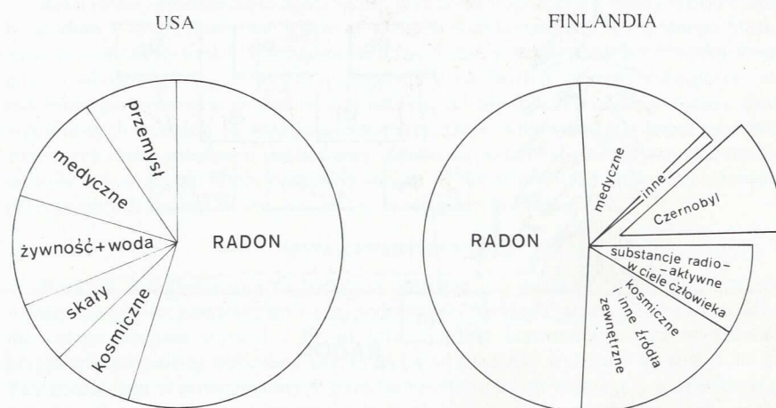
Rys. 1. Przykłady efektywnego równoważnika dawki promieniowania jonizującego otrzymywanego przez mieszkańca USA i Finlandii
