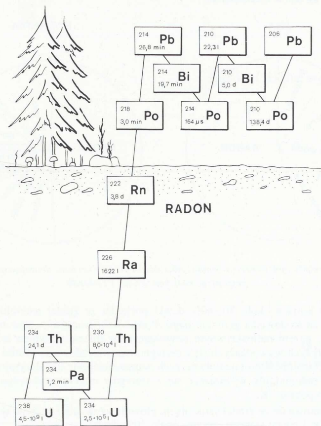
Rys. 2. Schemat przemian promieniotwórczych szeregu uranowo-radowego [5]
